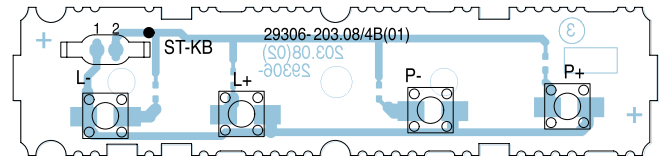
Ansicht von der Bestückungsseite / View of Component Side
