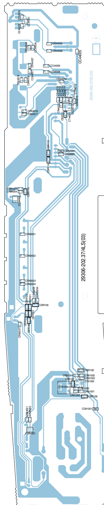
Ansicht von der Lötseite / View of Solder Side
