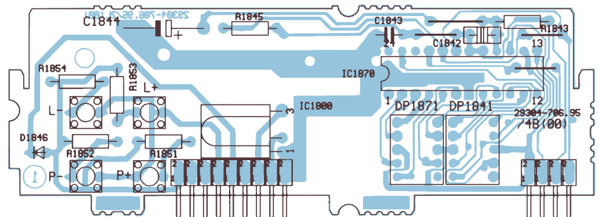
Ansicht von der Bestückungsseite / View of Component Side
