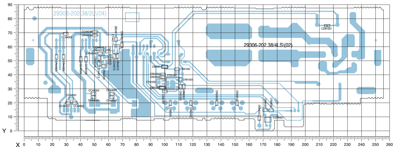
Ansicht von der Lötseite / View of Solder Side
